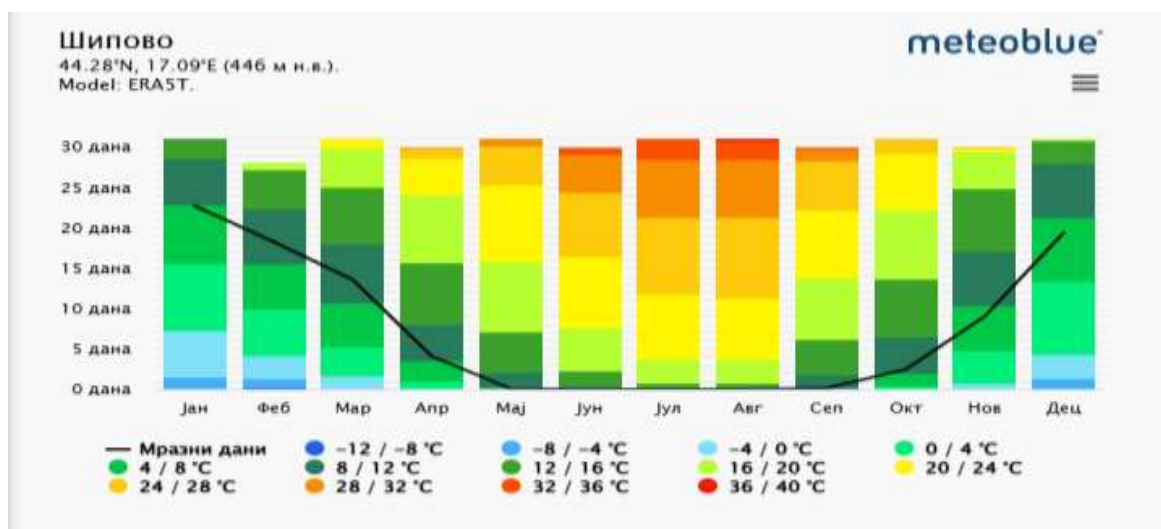
Slika br.5. Maksimalne temperature u opštini Šipovo ( www.meteoblue.com )
