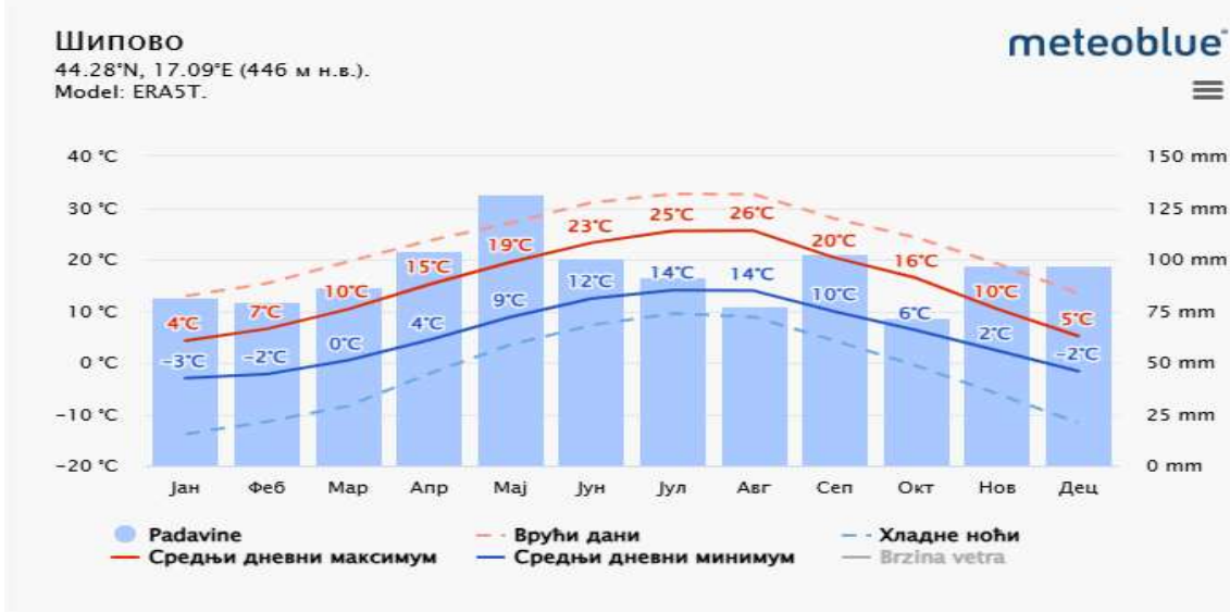
Slika br.3. Prosječne temperature i padavine u opštini Šipovo ( www.meteoblue.com )
